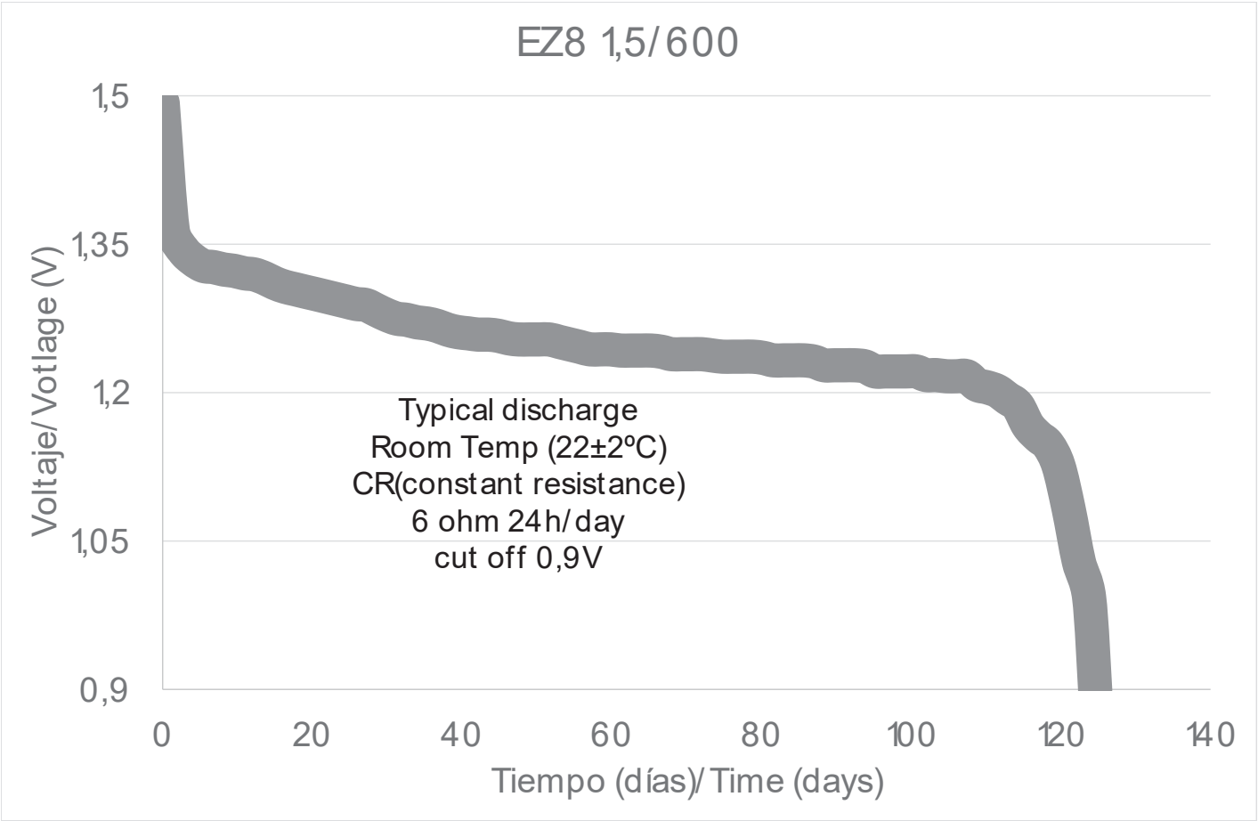
DURÉE DE VIE DE LA BATTERIE E/Z8 1,5/600 BASÉE SUR UNE DÉCHARGE CONTINUE MOYENNE ET UNE UTILISATION 24 H/JOUR
