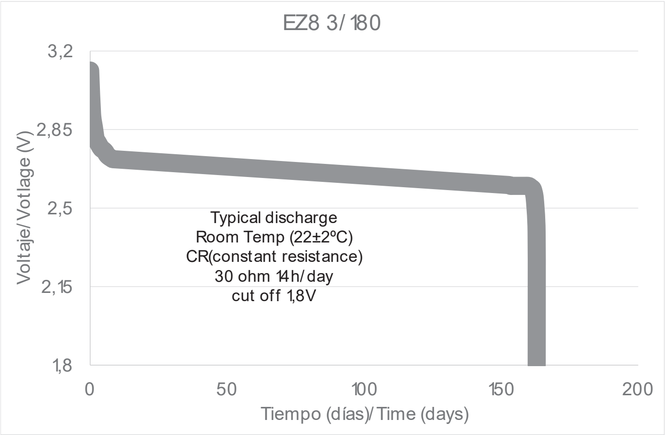
DURÉE DE VIE DE LA BATTERIE E/Z8 3/180 BASÉE SUR UNE DÉCHARGE CONTINUE MOYENNE ET UNE UTILISATION 24 H/JOUR
