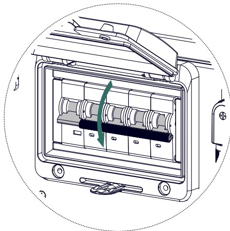
Abbildung 8-1 Deaktivieren Sie den Leistungsschalter (CB).
