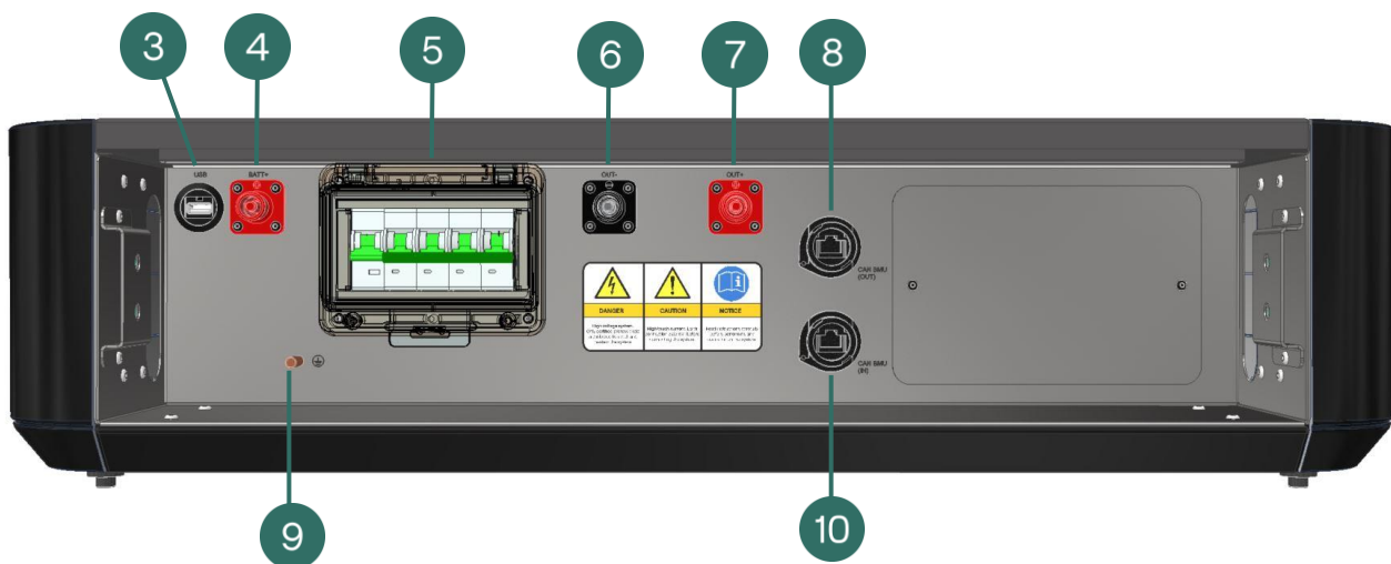
Abbildung 3-5 BMU Rückseite
