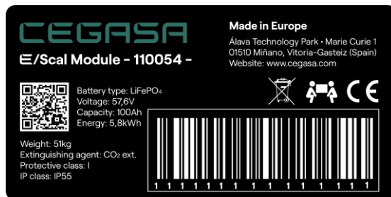
Abbildung 2-1 Modul E/Scal HV - Warnschild 1
