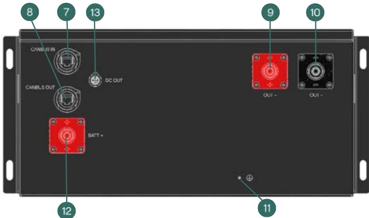
Abbildung 3-9 BMU Rückseite
