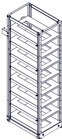
Abbildung 3-4 Struktur
