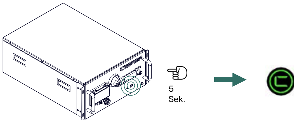
Abbildung 6-2 Systemstopp
