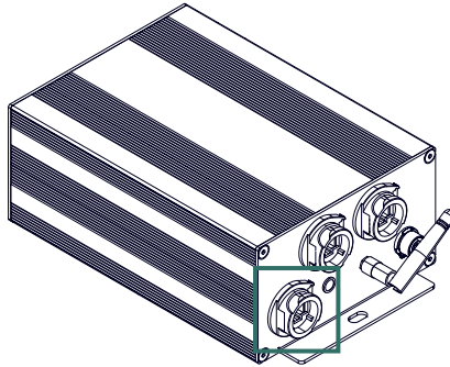
Abbildung 5-4 Master-Gerät Rückseite
